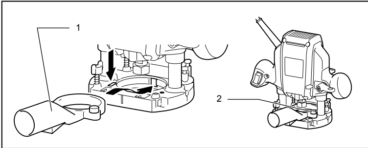
1. Absaugstutzen 2. Flügelschraube
